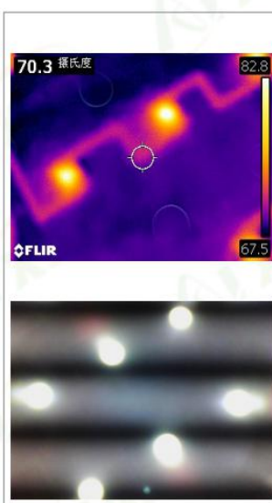
灯板(PCB)
