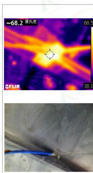
外壳(housing)
